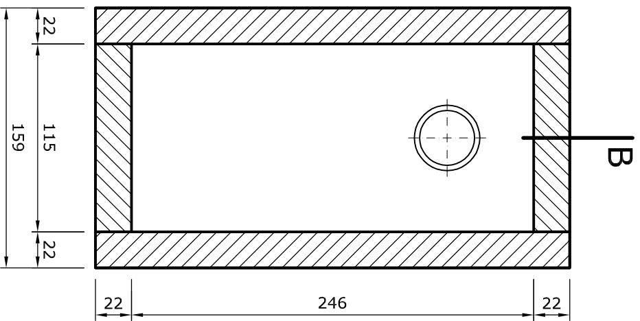
doorsnede A
