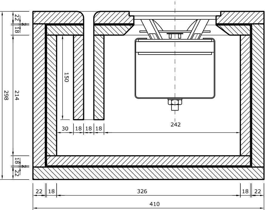
verticale doorsnede
