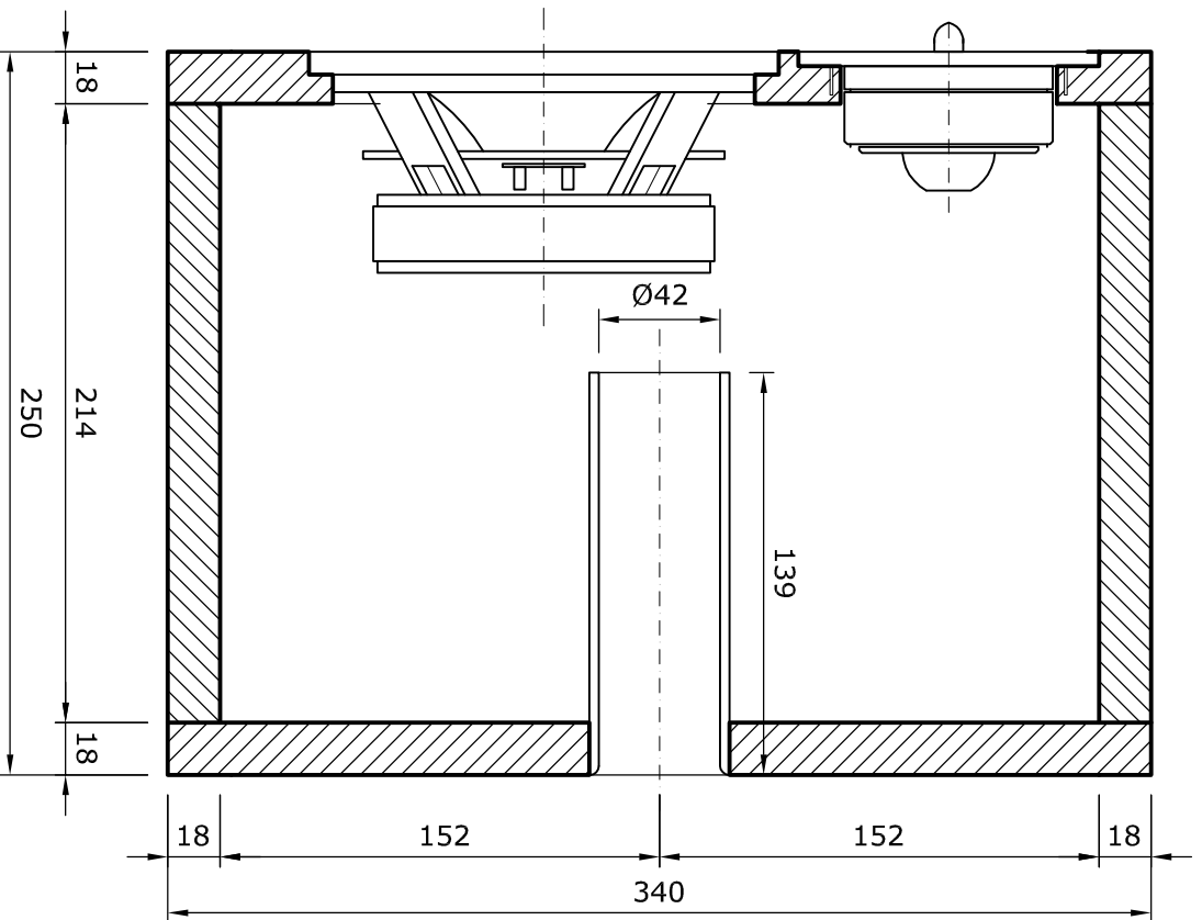
doorsnede B
