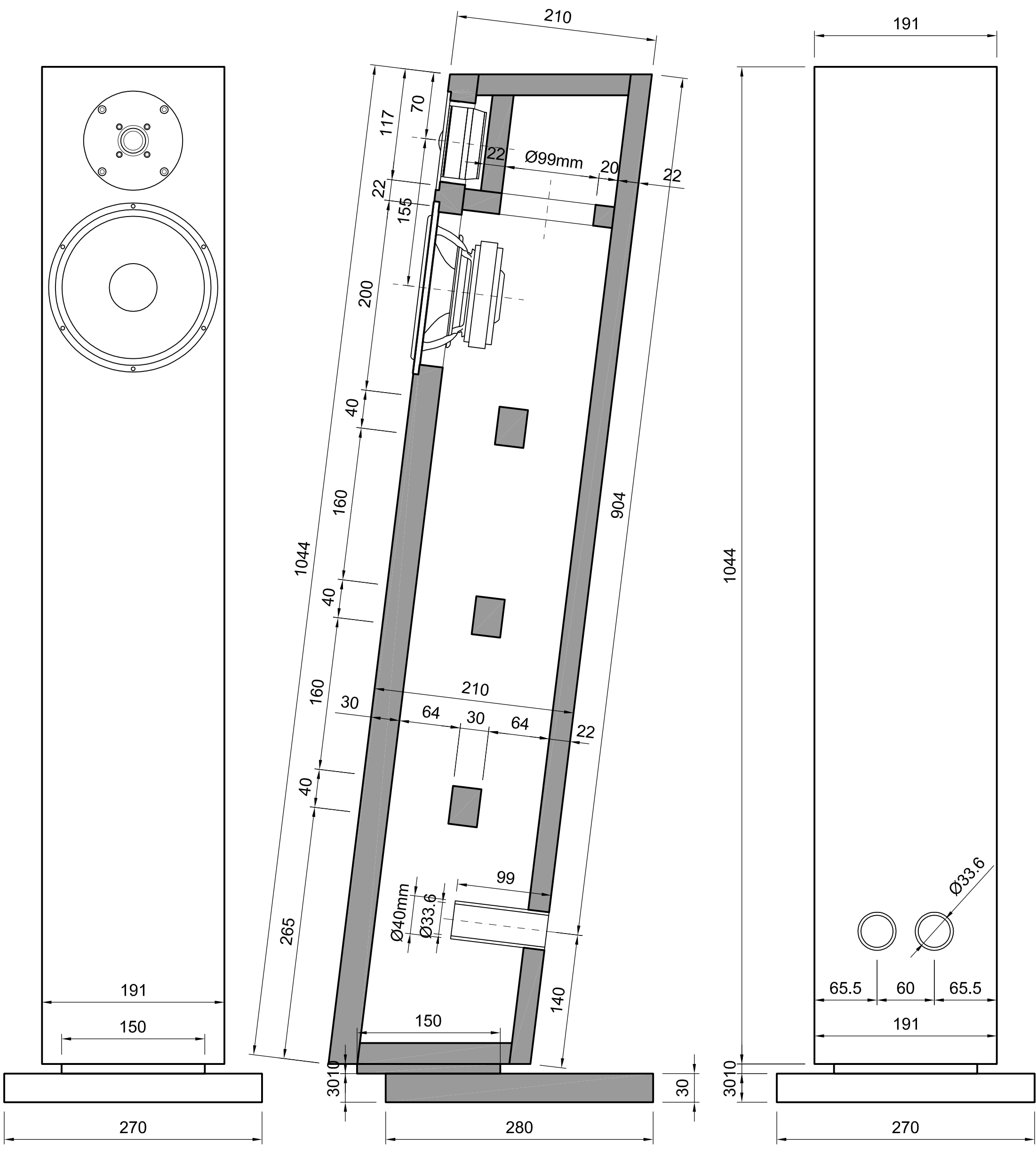
vooraanzicht
