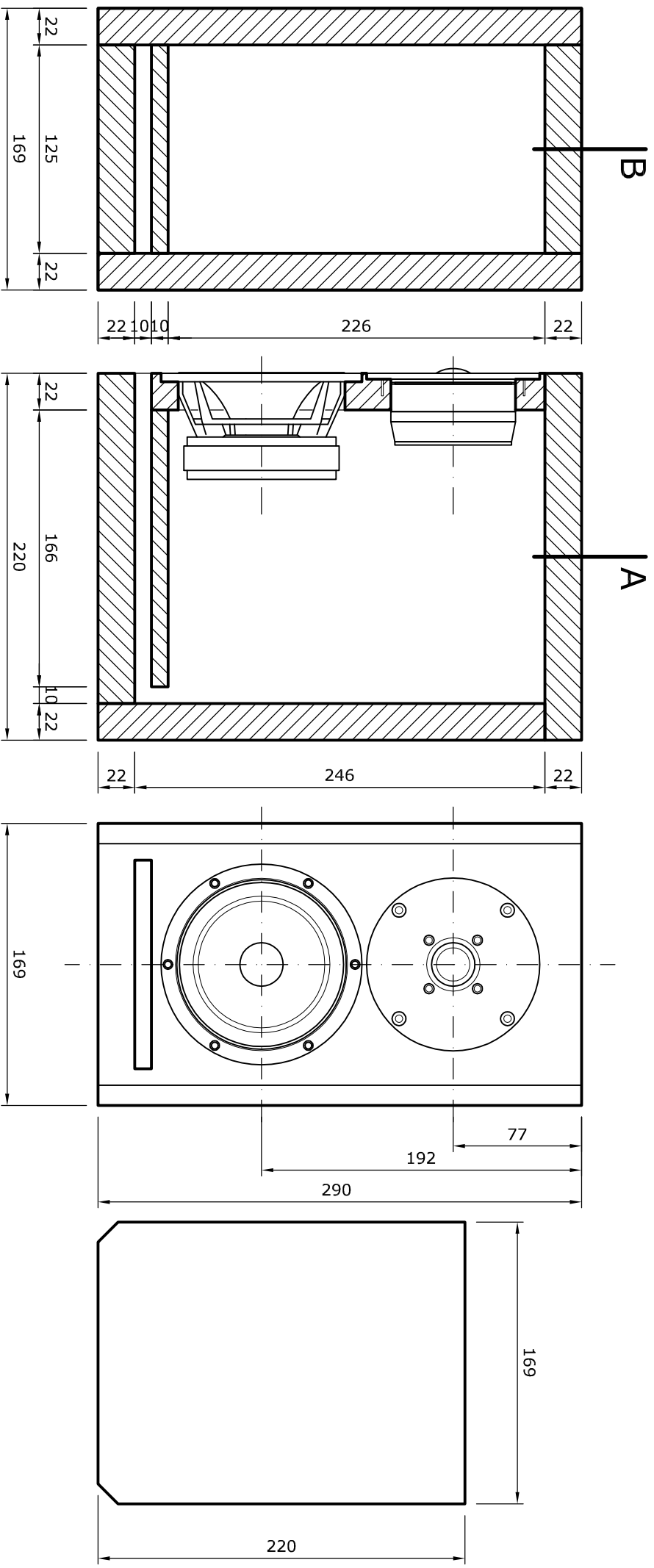
doorsnede A
