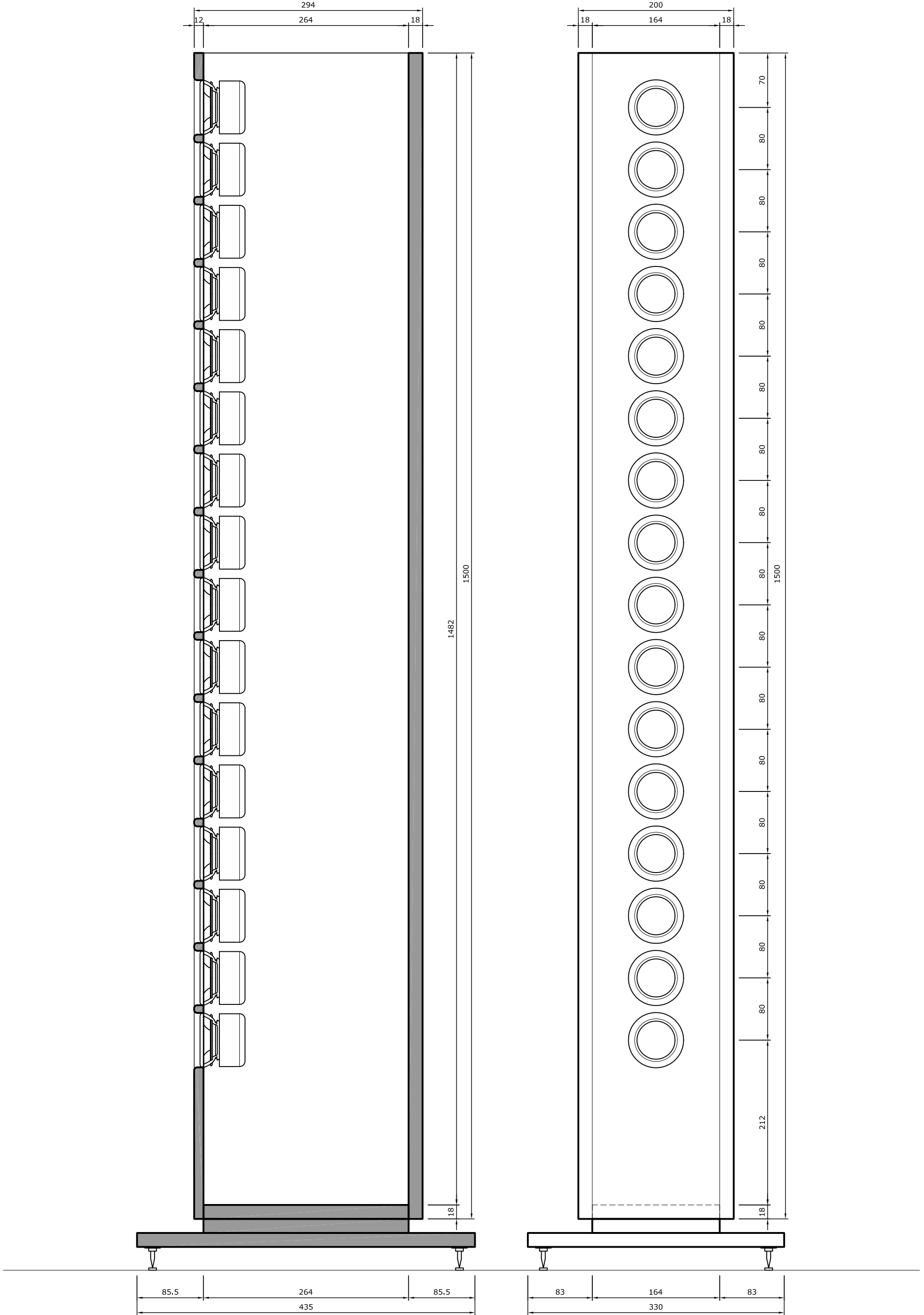
verticale doorsnede
