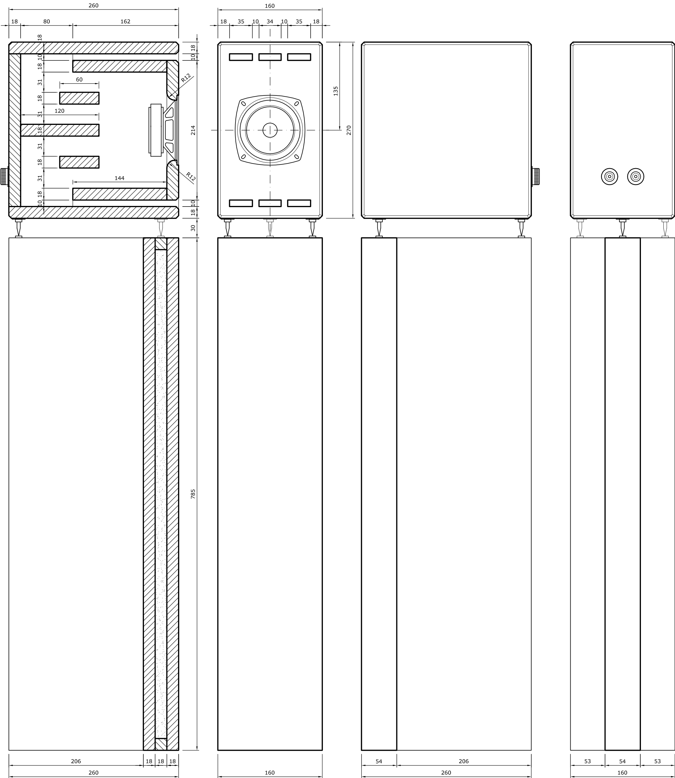
verticale doorsnede
